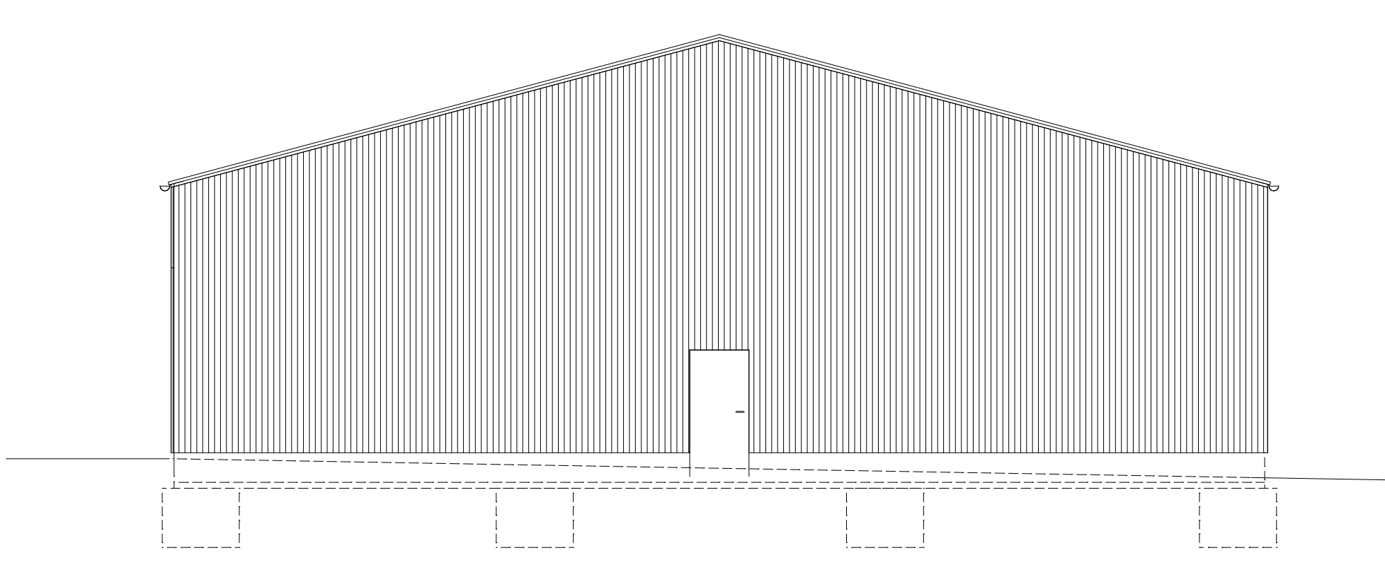
ANSICHT OST
